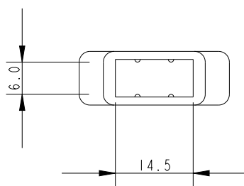
SECTION XSEC0001-XSEC0001 SCALE 1:1
